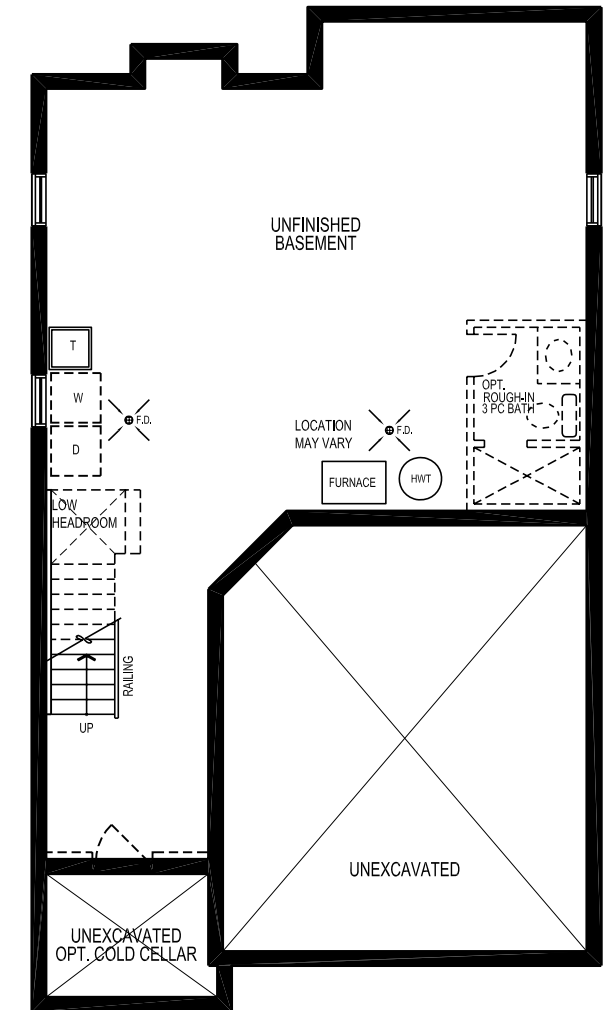
BASEMENT PLAN 'A' & 'B'
